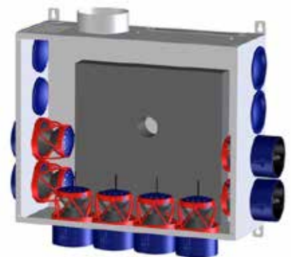
Een verdeelbox (plenum) met regelbare kleppen. Ieder afvoerpunt is met een apart ventilatiekanaal hierop aangesloten. Met de kleppen wordt de capaciteit per afvoerpunt geregeld.
